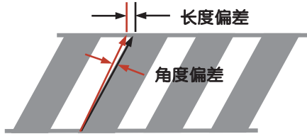
螺旋角偏差
