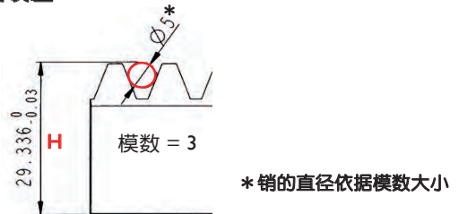
高度误差
